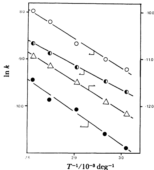
Fig. 2. Arrhenius plot.
